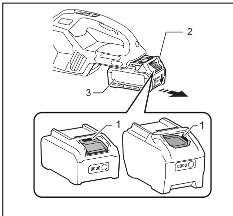
► 1. Indicateur rouge 2. Bouton 3. Batterie
