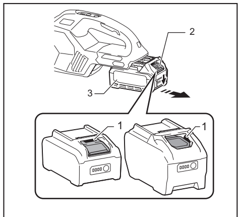
► 1. Indicador rojo 2. Botón 3. Cartucho de batería
