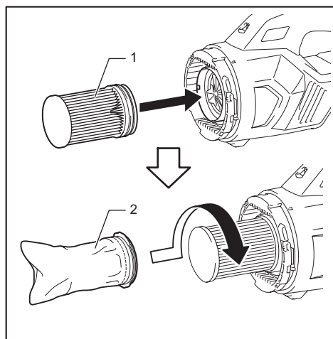
► 1. Filtre HEPA 2. Filtre haute performance
