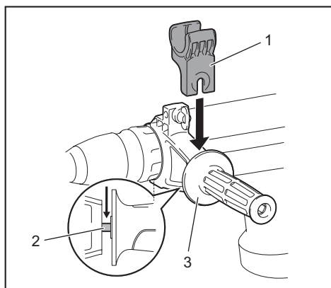
► 1. Support de tuyau 2. Arbre 3. Poignée latérale
