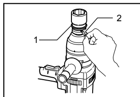
1. Anillo-O 2. Clavija
