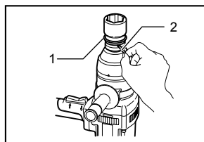
1. Joint torique 2. Broche
